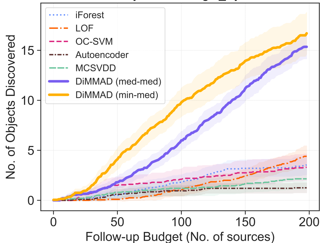
Anomaly: uLens-Single_PyLIMA
